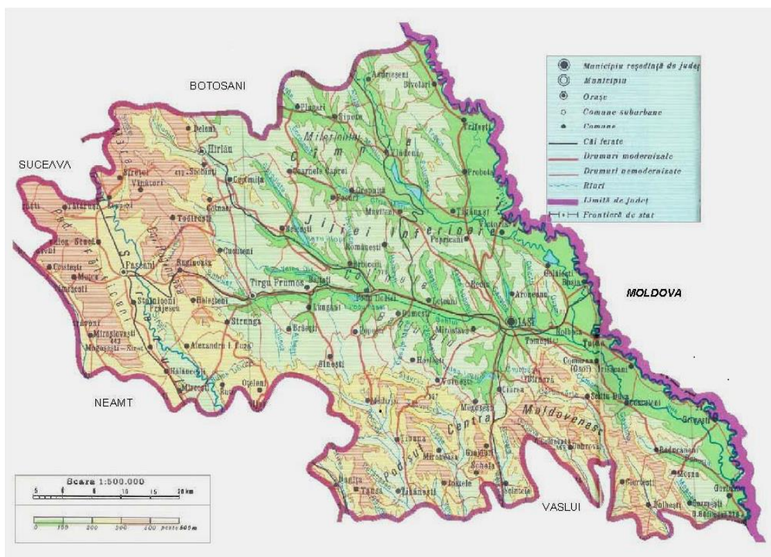
Fig. 2.2.2 Geologie - comuna Răchiteni, județul Iași
