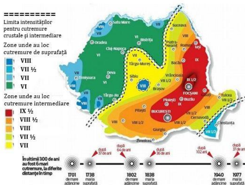
Fig 2.4.1 Harta riscului seismic
