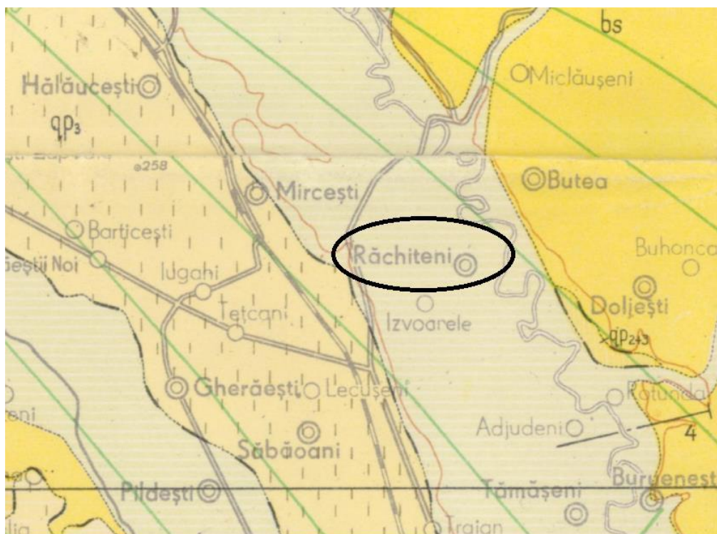
Fig. 2.2.3 Geologie – comuna Răchiteni, județul Iași
